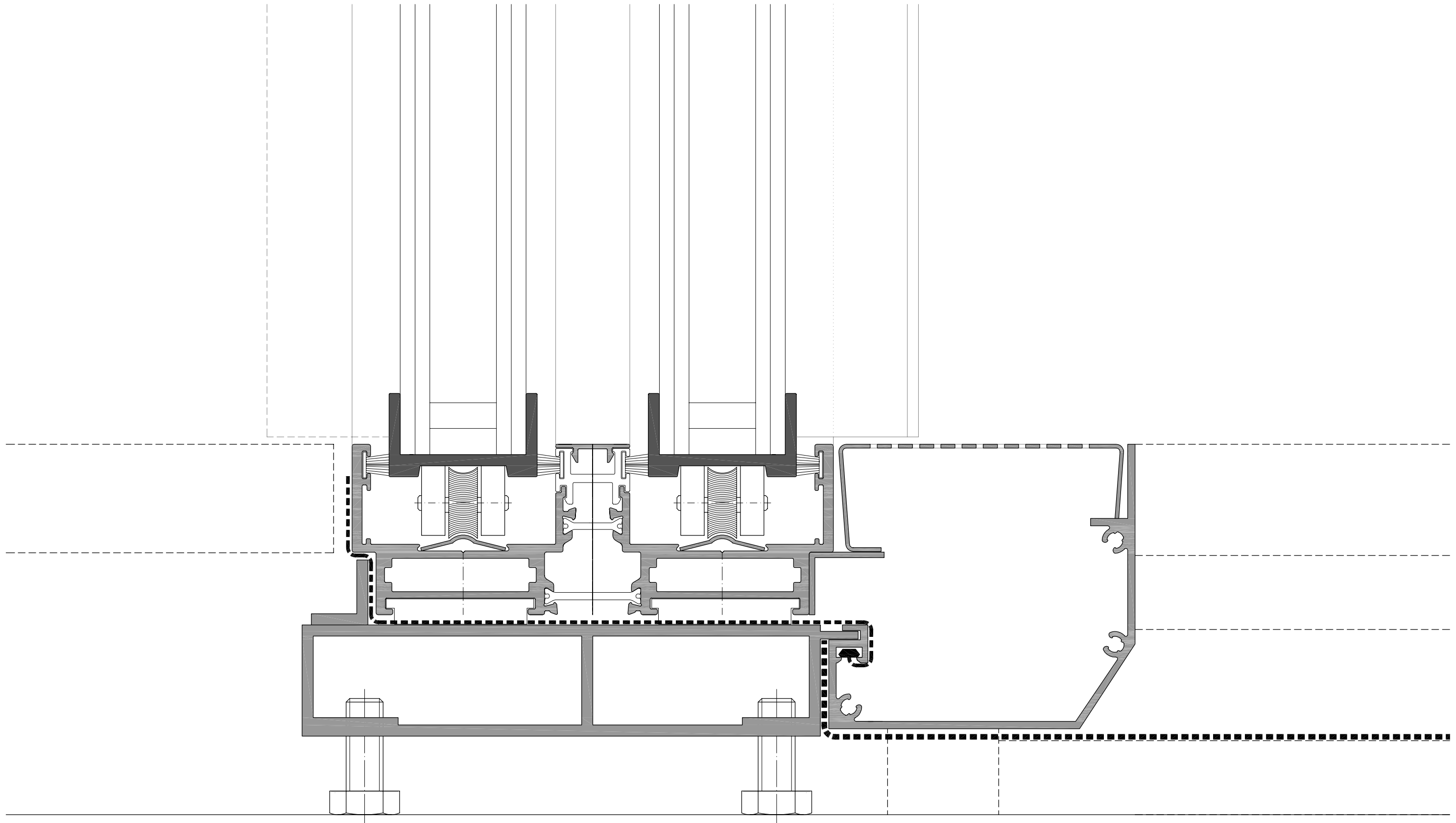
DETALLE DRENAJE
